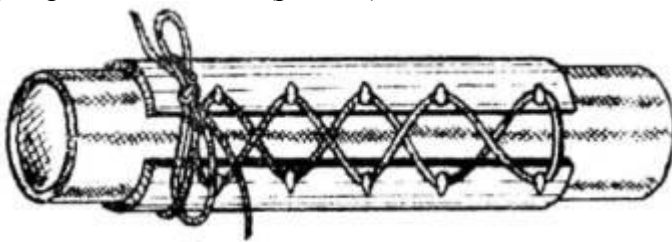
Рис. 10. Корсетный зажим
